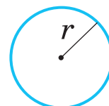
Окружность C = 2\pi r
