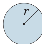
Круг S = \pi r^2
