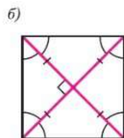
Свойства квадрата
