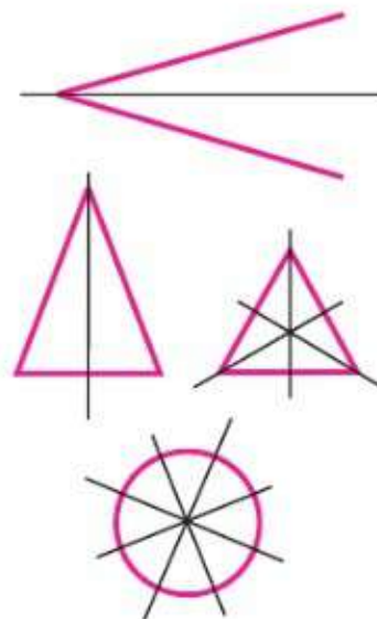
Фигуры, обладающие осевой симметрией
