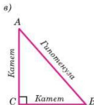
Прямоугольный треугольник
