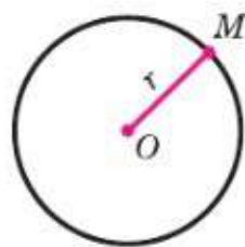
Окружность радиуса r с центром O
