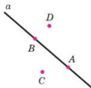
Прямая и точки
