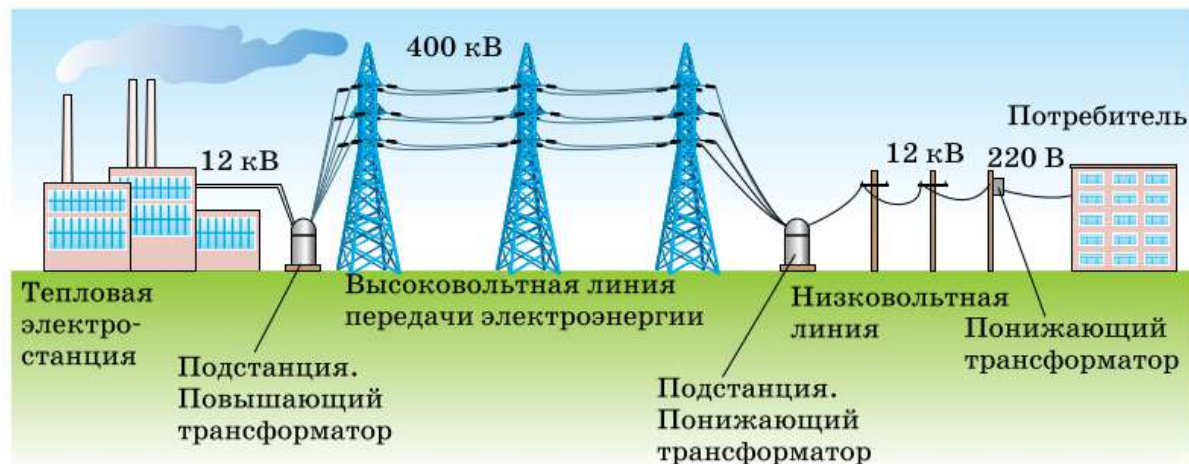
Рис. 177. Схема передачи электроэнергии от электростанции к потребителю
