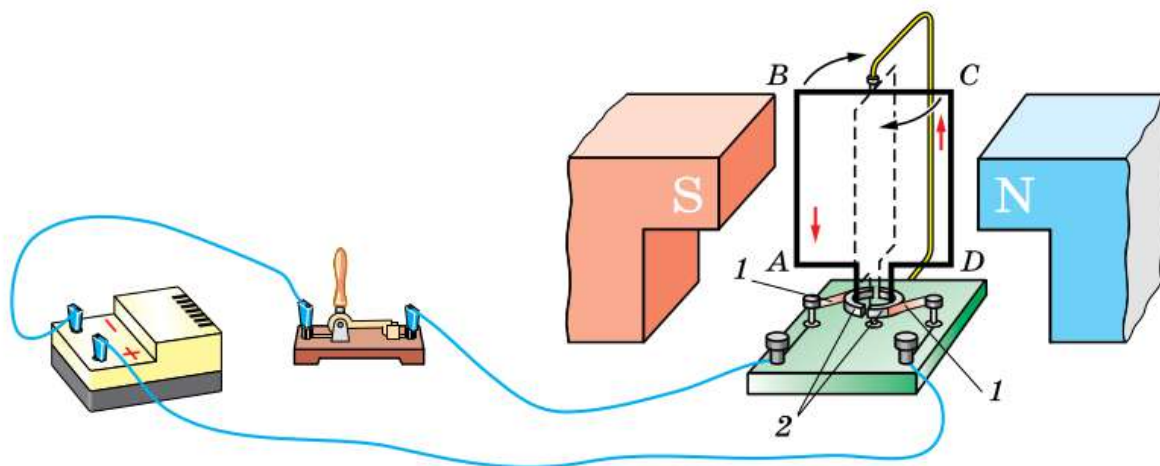
Рис. 159. Вращение рамки с током в магнитном поле
