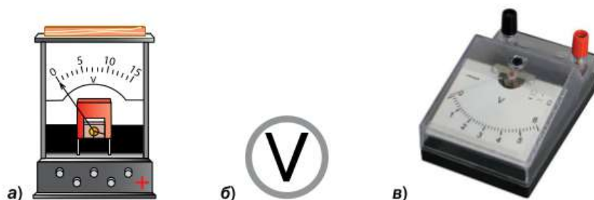
Рис. 95. Вольтметр: а — демонстрационный; б — условное обозначение на схемах; в — лабораторный
