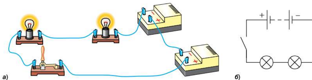
Рис. 106. Последовательное включение электрических ламп и источников тока
