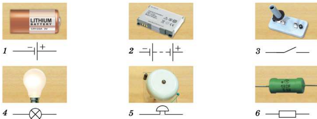
Рис. 78. Условные обозначения, применяемые на схемах:
