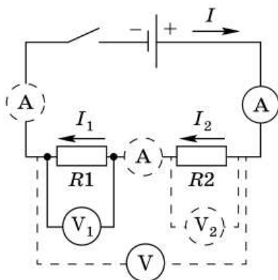
Рис. 107. Последовательное соединение проводников
