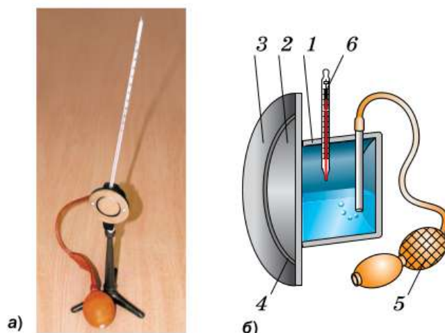
Рис. 39. Конденсационный гигрометр: а — внешний вид; б — устройство
