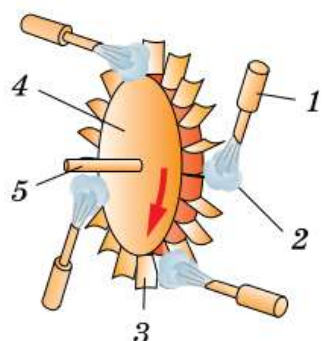
Рис. 51. Схема паровой турбины
