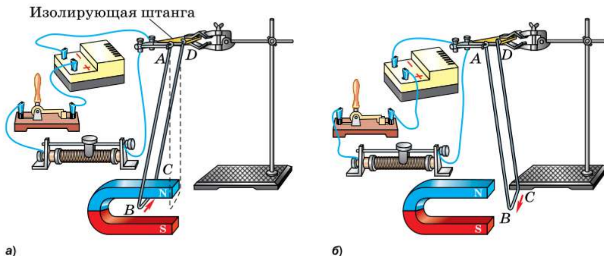
Рис. 144. Действие магнитного поля на проводник с током
