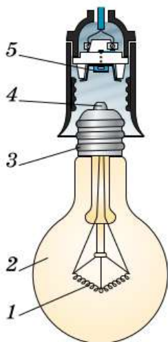
Рис. 110. Лампа накаливания:
