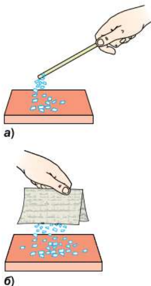
Рис. 53. Электризация трением
