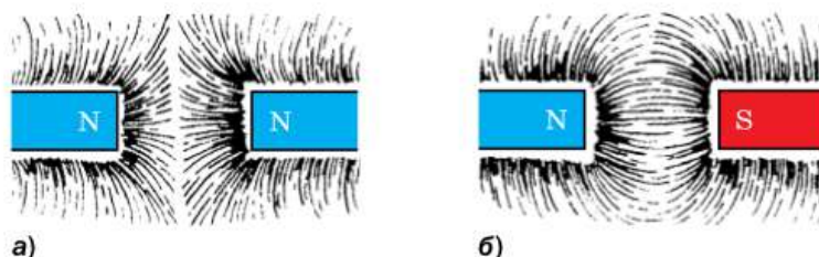
Рис. 128. Магнитные линии поля двух магнитов
