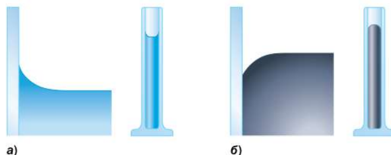
Рис. 5. Искривление поверхности жидкости вблизи стенок сосуда: а — смачивание; б — несмачивание
