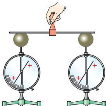
Рис. 65. Делимость электрического заряда
