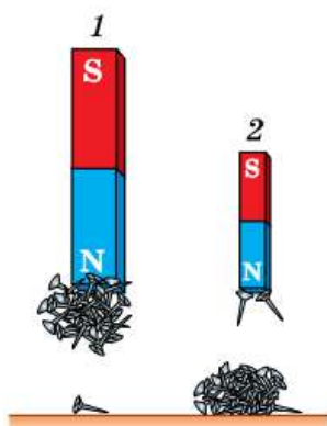
Рис. 154. Магнитное поле первого магнита сильнее, чем второго
