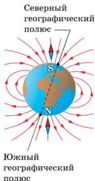
Рис. 142. Линии магнитного поля Земли
