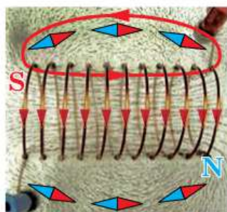
Рис. 132. Магнитные линии катушки с током
