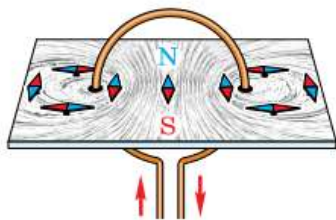
Рис. 125. Картина магнитного поля кругового витка с током
