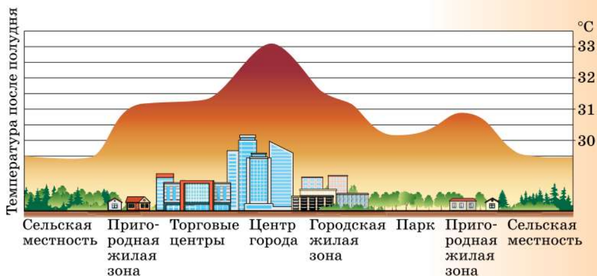
Рис. 23. Городской «остров тепла»
