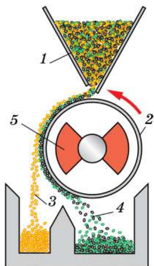
Рис. 138. Магнитный сепаратор
