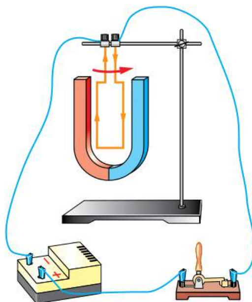
Рис. 86. Рамка с током между полюсами магнита поворачивается
