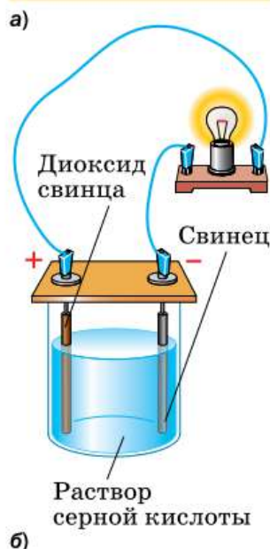
Рис. 76. Аккумулятор: а — внешний вид; б — принцип действия
