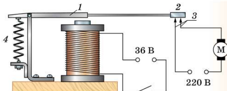
Рис. 141. Устройство реле
