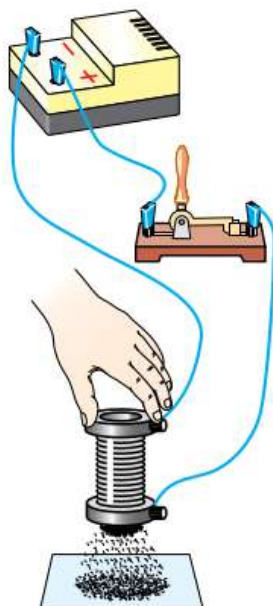
Рис. 131. Притяжение железных опилок катушкой с током
