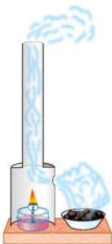
Рис. 20. Модель для демонстрации тяги
