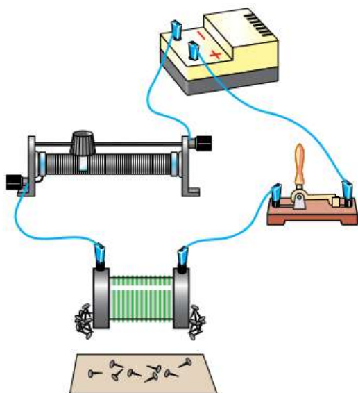
Рис. 134. Действие магнитного поля катушки
