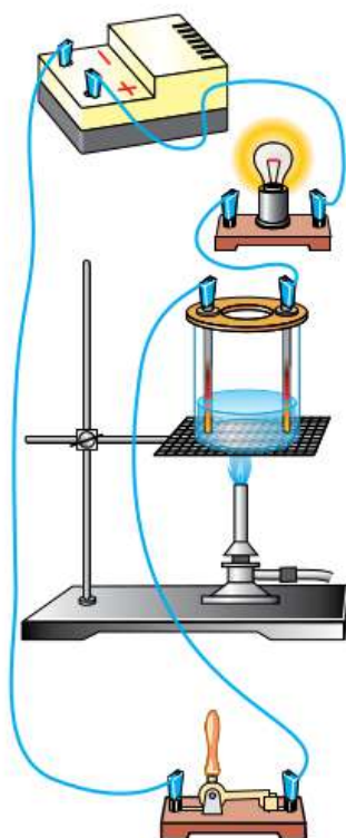
Рис. 83. Химическое действие тока
