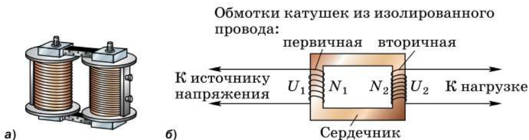
Рис. 176. Повышающий трансформатор: а — внешний вид; б — схема устройства
