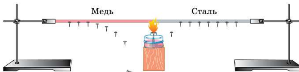
Рис. 15. Теплопроводность разных веществ
