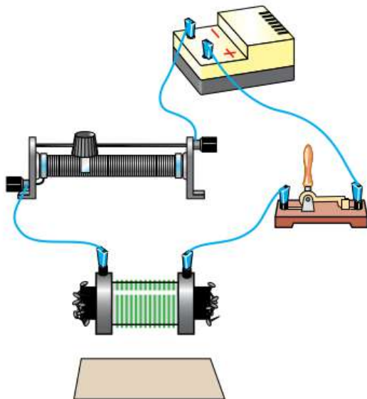
Рис. 135. Действие магнитного поля катушки с железным сердечником
