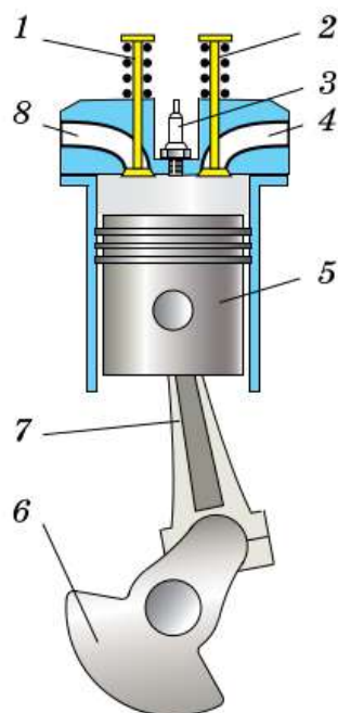
Рис. 48. Двигатель внутреннего сгорания (карбюраторный) в разрезе
