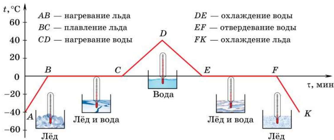
Рис. 31. График зависимости температуры льда от времени нагревания
