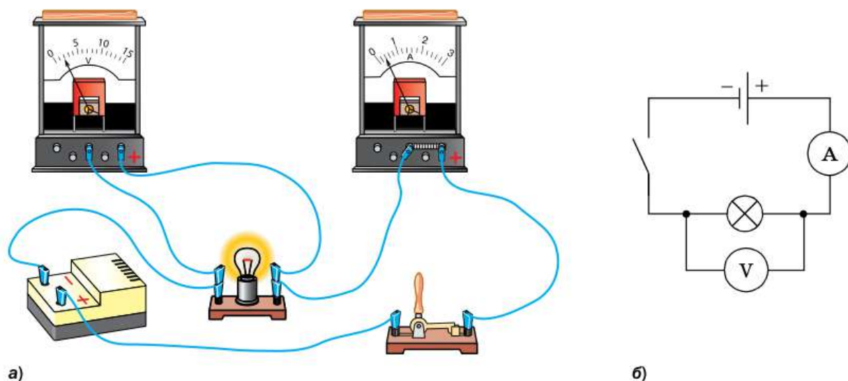
Рис. 96. Подключение вольтметра и амперметра в цепь
