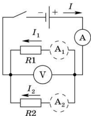
Рис. 109. Параллельное соединение проводников
