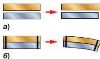
Рис. 115. При нагревании биметаллическая пластина изгибается
