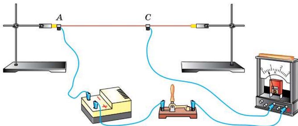
Рис. 104. Изменение длины проводника, включённого в электрическую цепь
