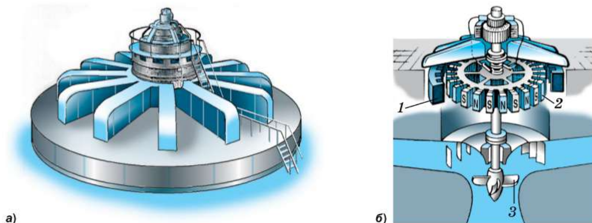
Рис. 174. Внешний вид (а) и устройство (б) мощного гидрогенератора
