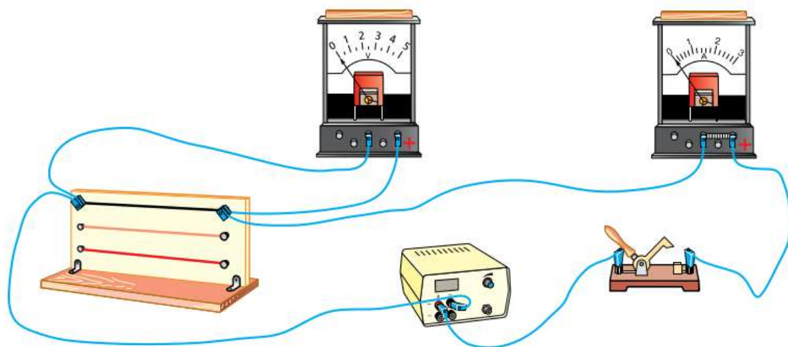
Рис. 98. Определение зависимости силы тока от напряжения
