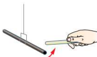
Рис. 55. Притяжение наэлектризованных эбонитовой и стеклянной палочек
