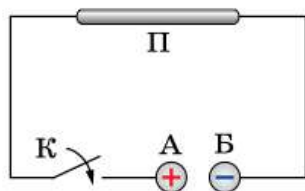
Рис. 71. Протекание электрического тока по проводнику
