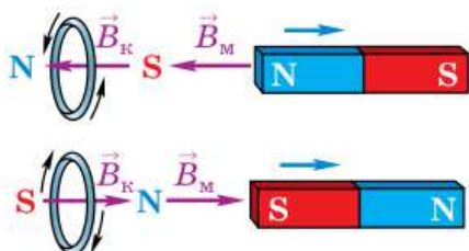
Рис. 172. Направление индукционного тока в кольце меняется при изменении направления движения магнита относительно кольца
