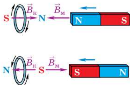
Рис. 170. Определение направления индукционного тока в кольце
