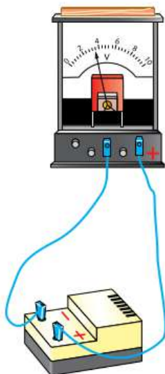
Рис. 97. Подключение вольтметра к источнику тока
