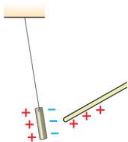
Рис. 68. Притяжение незаряженной гильзы к заряженной палочке
