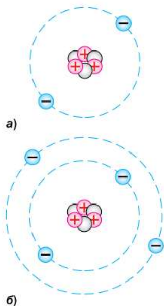
Рис. 67. Ион лития: а — положительный; б — отрицательный
