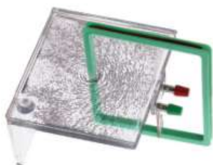
Рис. 122. Картина магнитного поля прямого проводника с током
