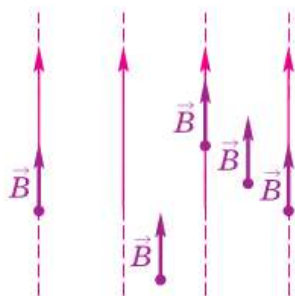
Рис. 157. Однородное магнитное поле
