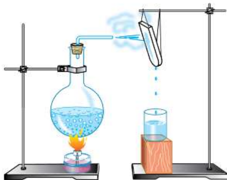
Рис. 44. Конденсация пара
