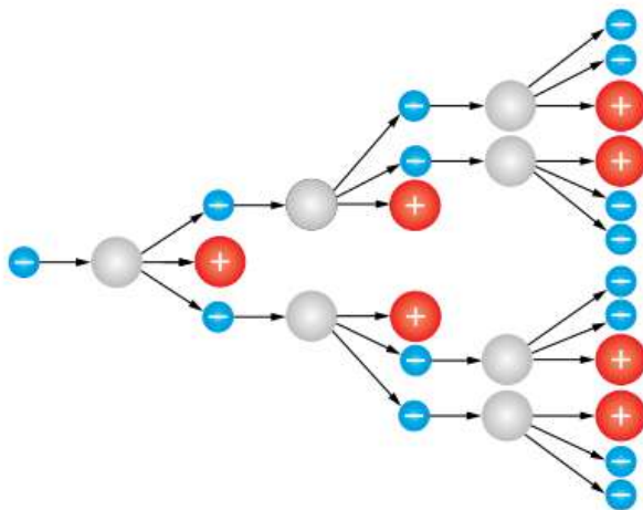
Рис. 111. Лавинообразное увеличение числа свободных заряженных частиц
