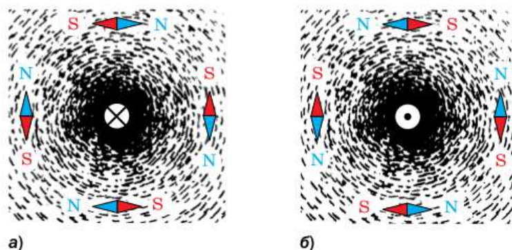
Рис. 123. Расположение магнитных стрелок вокруг проводника с током
