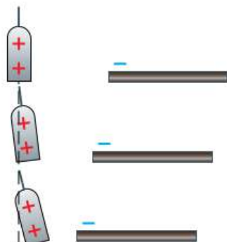
Рис. 61. Чем ближе друг к другу заряженные тела, тем сильнее их взаимодействие
