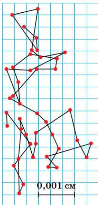
Рис. 1. Положения броуновской частицы, отмеченные через каждые 30 с
