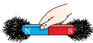
Рис. 118. Полюсы магнита
