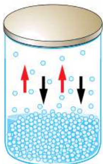
Рис. 34. Испарение жидкости в закрытом сосуде
