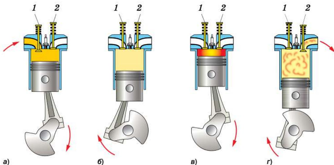
Рис. 49. Циклы работы двигателя внутреннего сгорания (карбюраторного)
